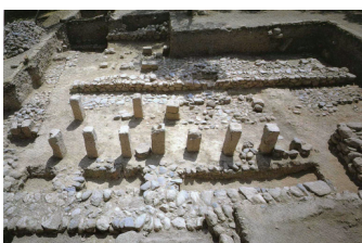
上層の列柱式建物
